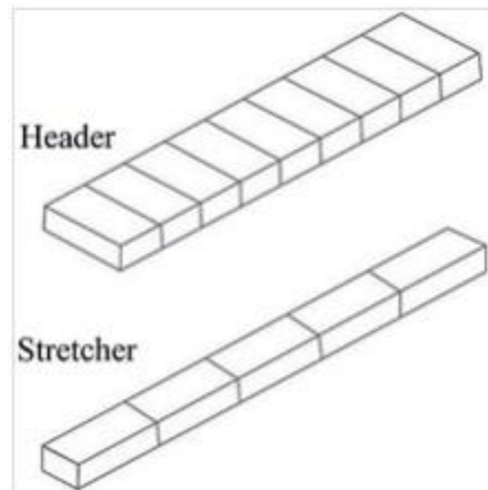
Alineamientos de ladrillos de frente («header») y extendido («stretcher») utilizados en la construcción.
